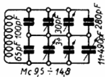
CIRCUITO D'ANTENNA
