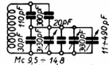
CIRCUITO OSCILLANTE
